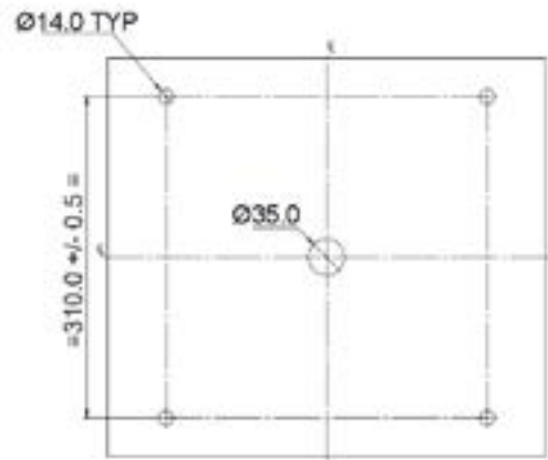
Anordnung der Montagebohrungen – Abmessungen in mm
