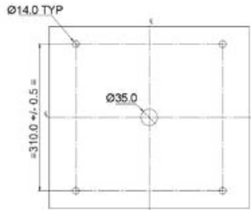
Disposizione dei fori di montaggio - dimensioni in mm.
