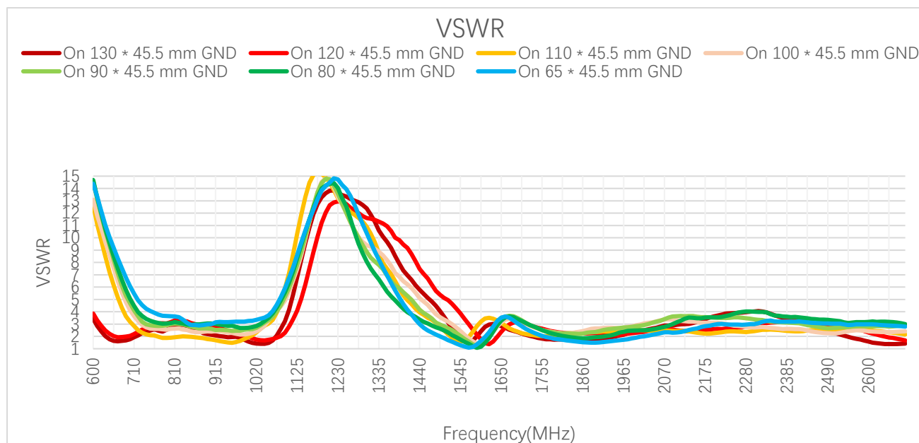
VSWR
