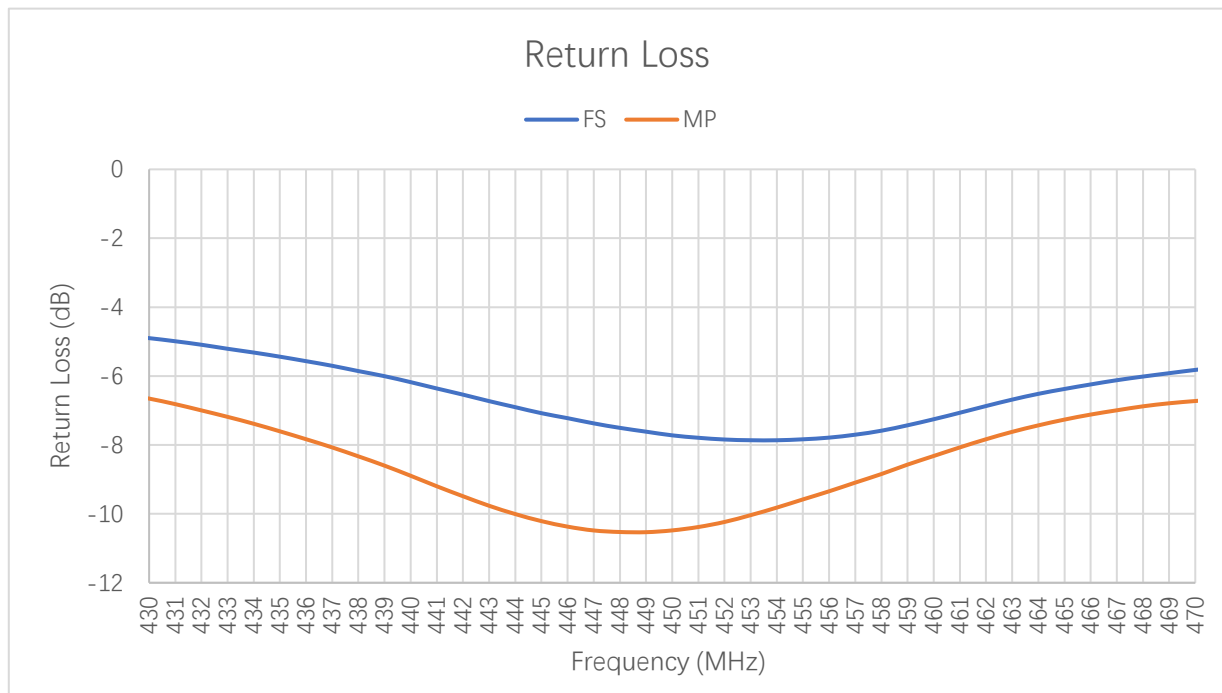
Return Loss(dB)
