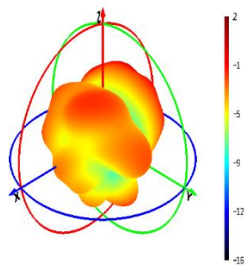
2450 MHz
