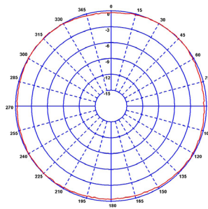
H-Plane (450MHz)
