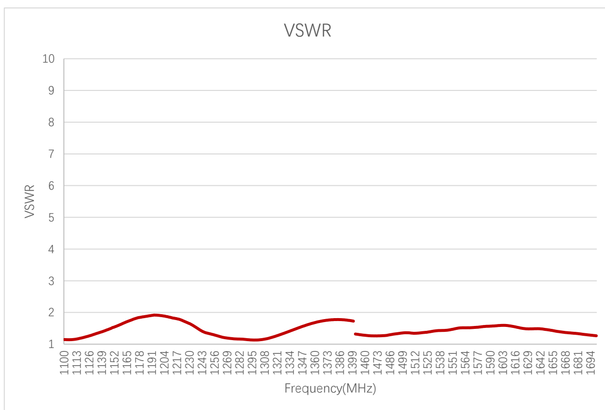
VSWR
